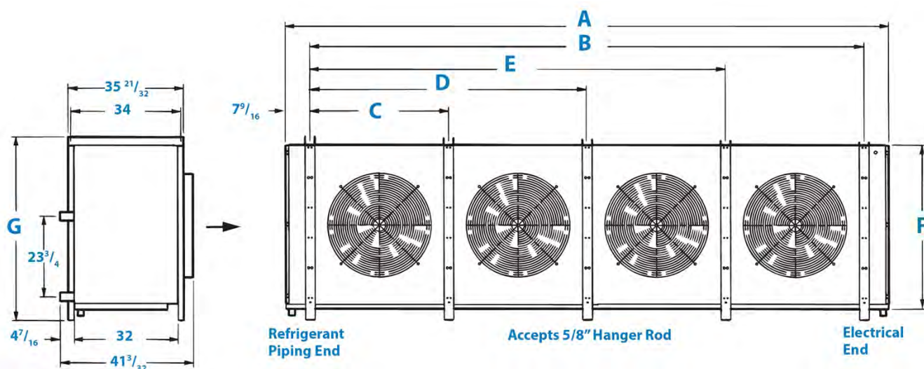
Diagram 2: 30" Fan Models"
